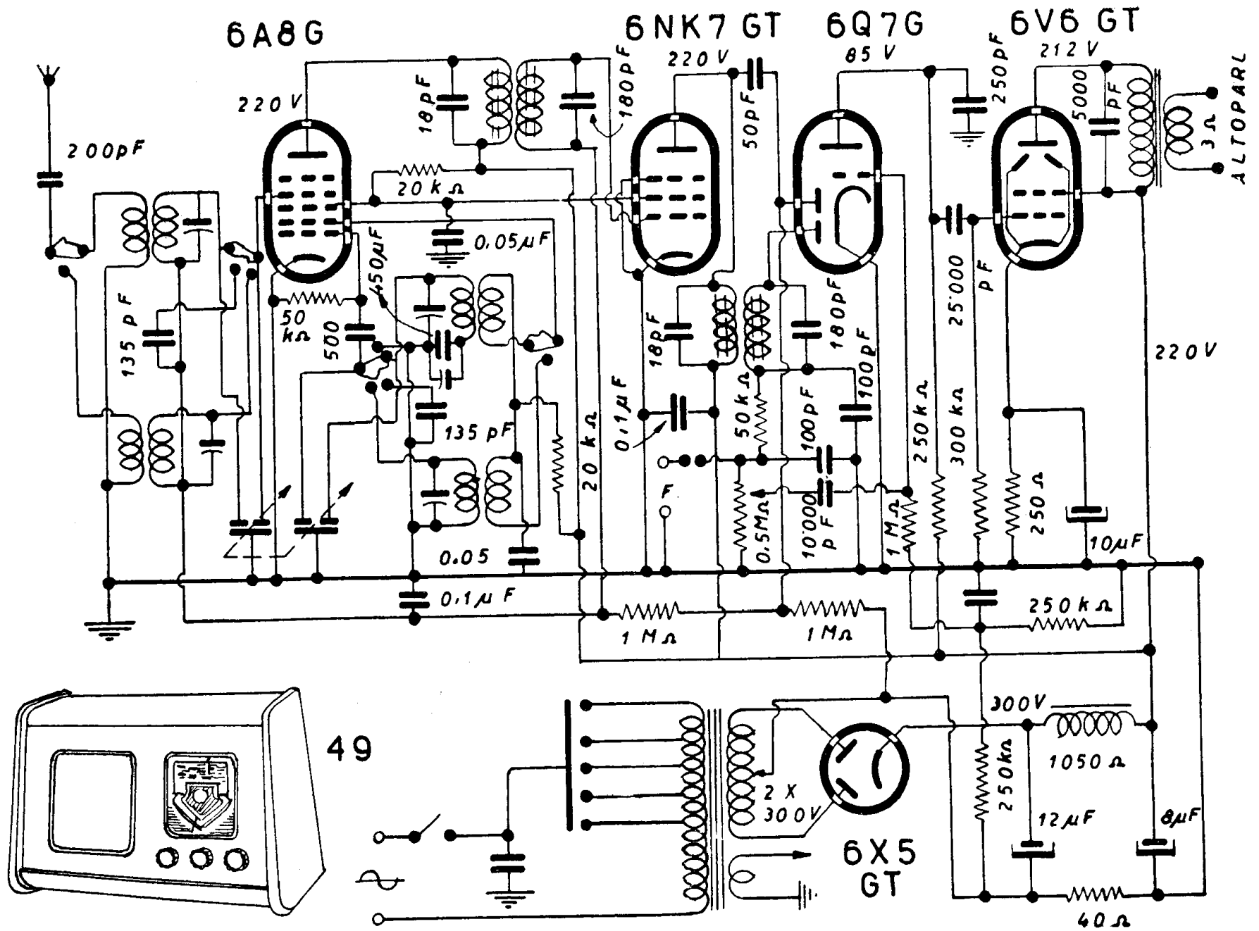
WATT RADIO - Mod. WATT 49 - Gamma medie da 580 a 188 m, corte da 50 a 37 m, cortissime da 37 a 18 m. Media frequenza 460 kc. Sensibilità di potenza 0,13 mV. Potenza d'uscita 4 W.
